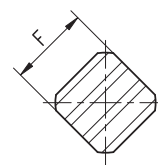
Corte AA (Quadrado de arraste)
