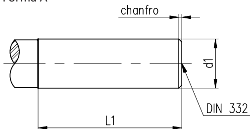
Forma A
